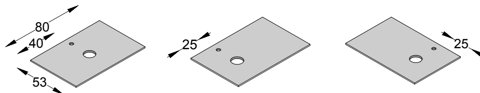
Art. KFU80 ct
